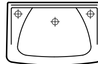
45cm basin W 45.5cm D 30.2cm H 21.7cm
