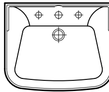
55cm basin W 55cm D 44cm H 85.5cm
