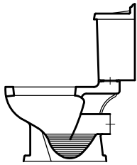
Close coupled wc suite W 35.6cm D 68.5cm H 82.5cm
