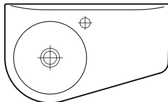
56cm side shelf basin W 56.2cm D 34cm H 17.5cm
