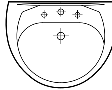
65cm basin W 65cm D 51.5cm H 85.5cm
